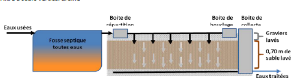
Filtre à sable vertical drainé
